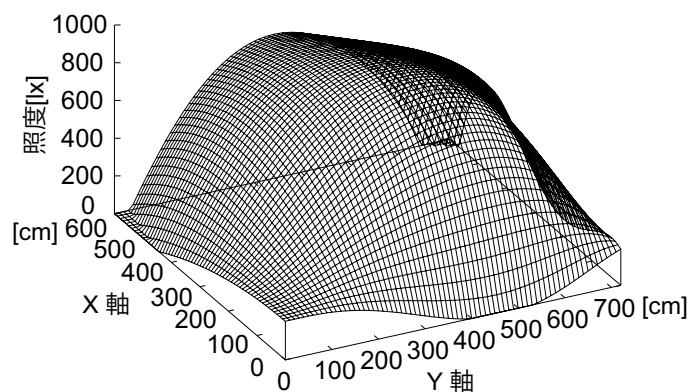
図 6: 提案手法で得られた照度分布図 (高さ 70 cm)
