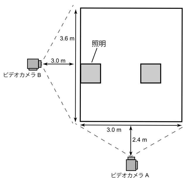
図 3: 実験環境の分割エリア (平面図)
